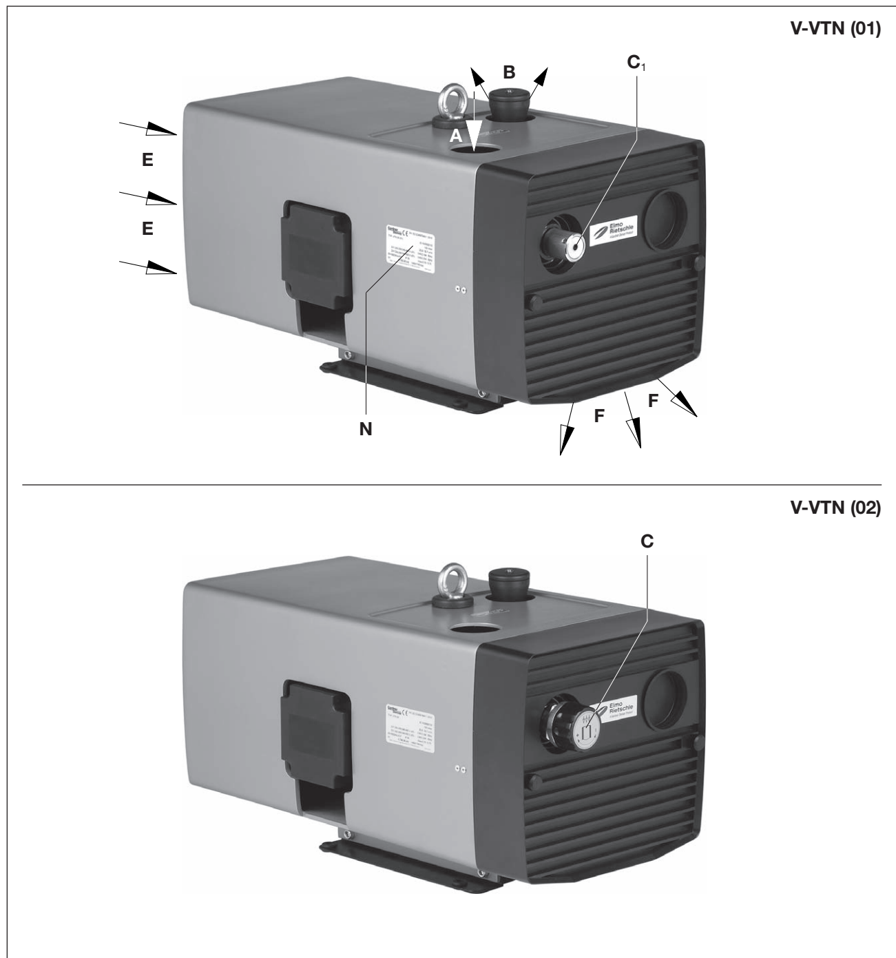
Abb. 2 Vakuumpumpe V-VTN (01) / V-VTN (02)
