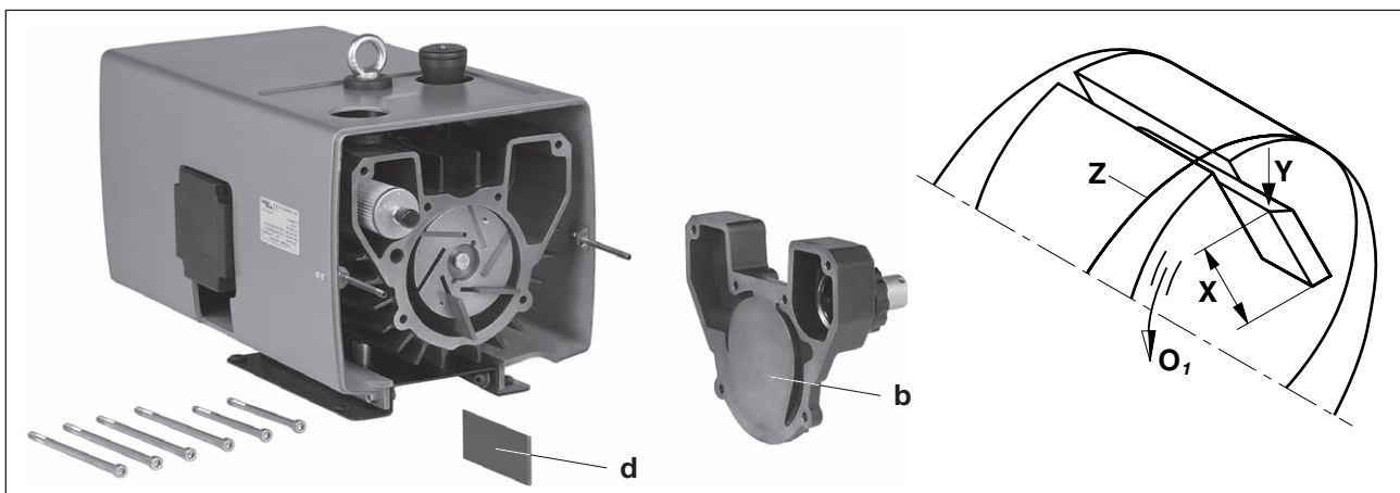
Abb. 7 Lamellenwechsel
