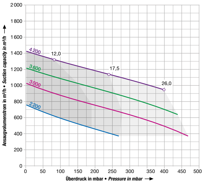
2BH1 940
