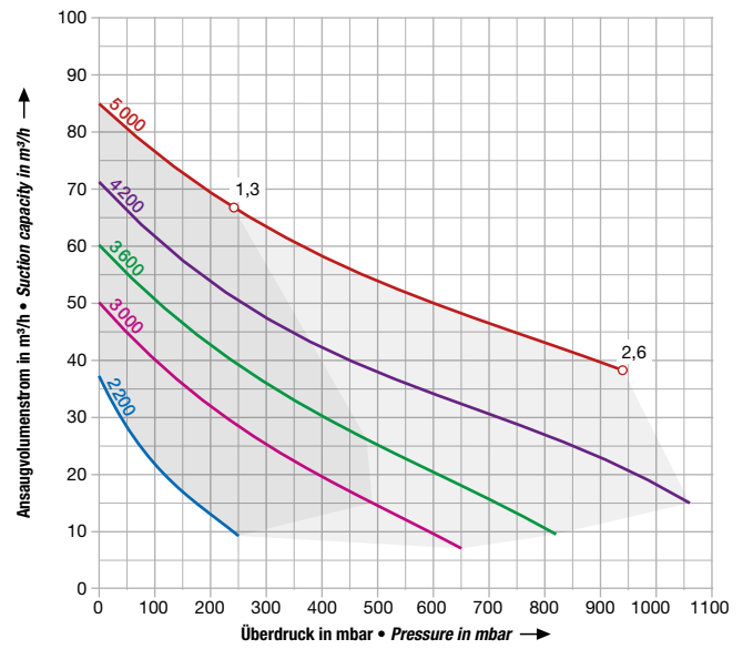
2BH7 320
