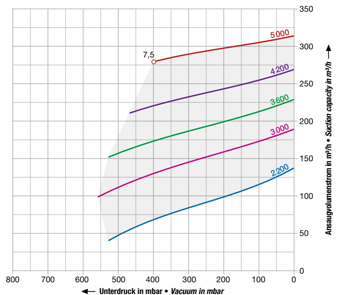
2BH7 630-0NN
