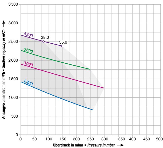
2BH9 2300
