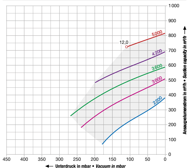
2BH1 830
