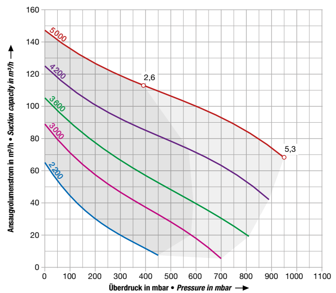
2BH7 420
