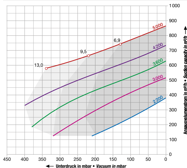
2BH1 840
