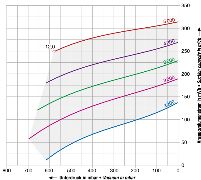
2BH7 630-0NH
