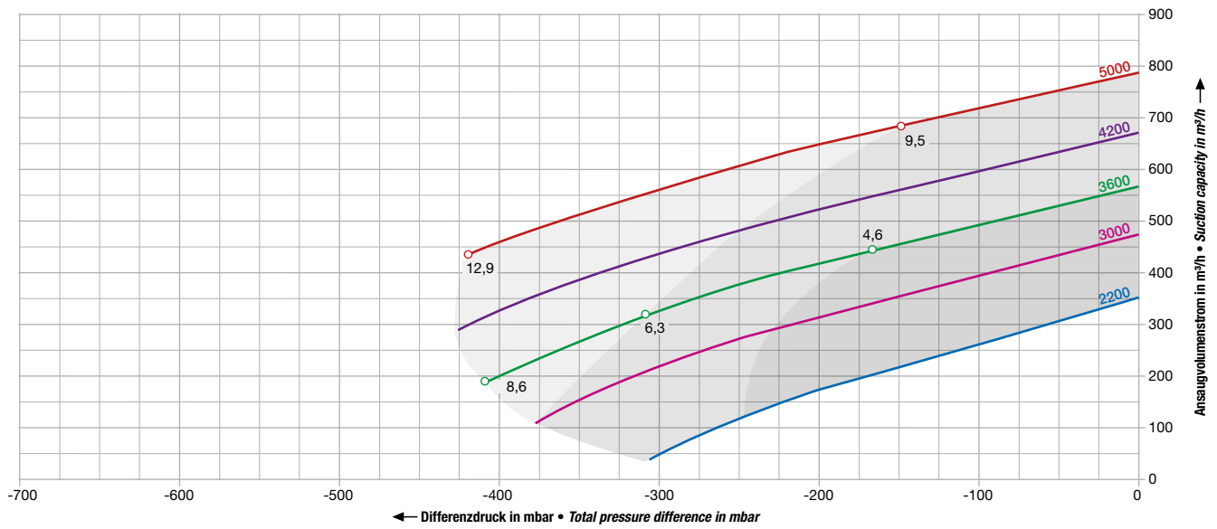
2BH2 0540 zweistufig • two stage
